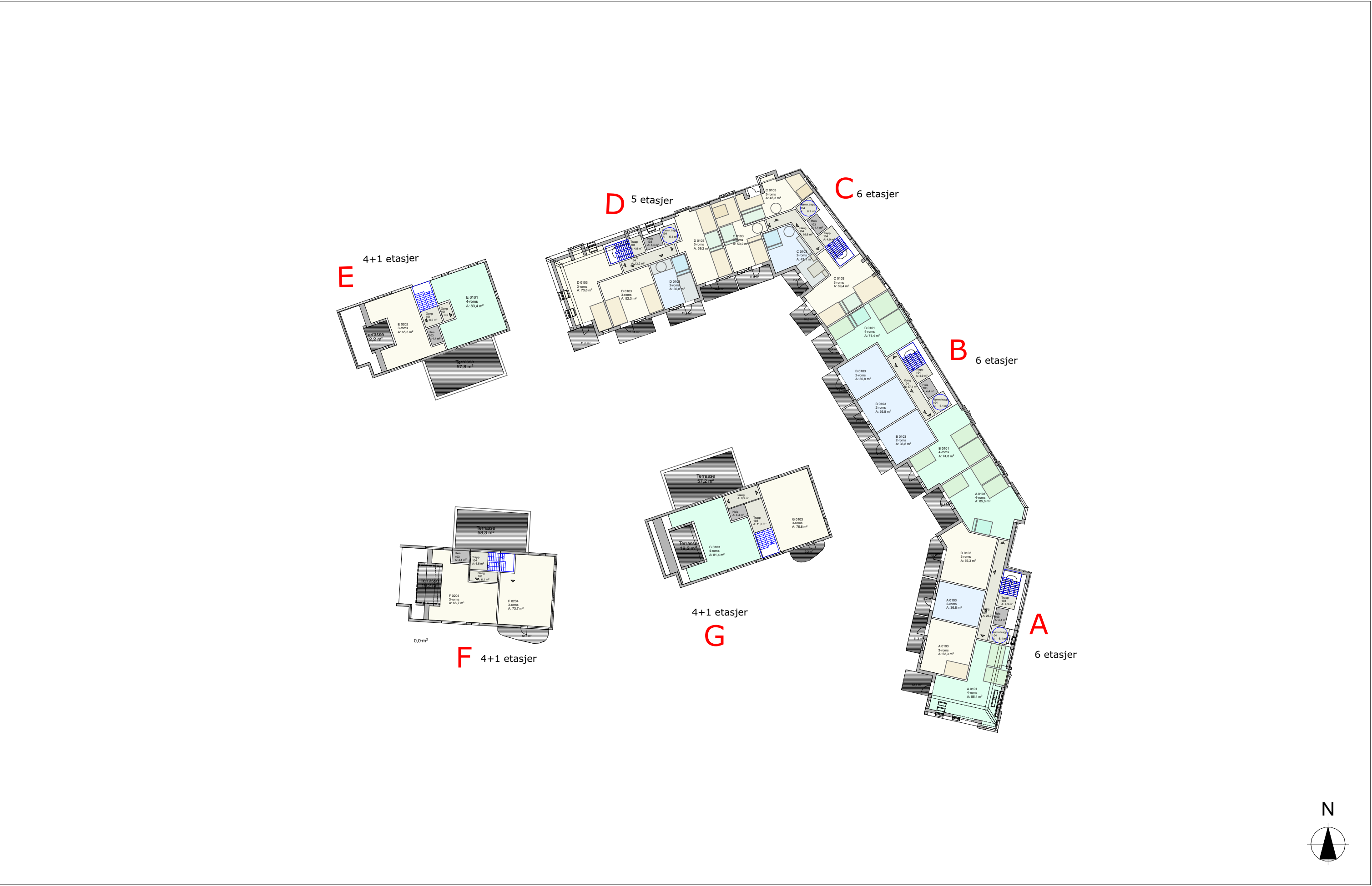
Plan 4. etasje
