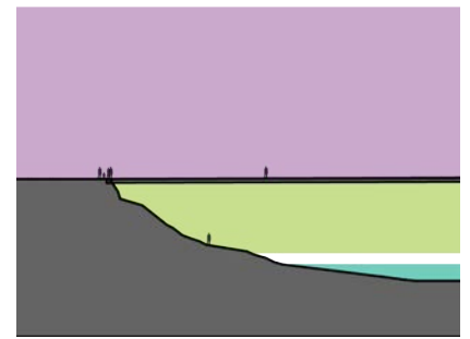
Øvre og nedre nivå. Snitt gjennom Elgeseter Bru
