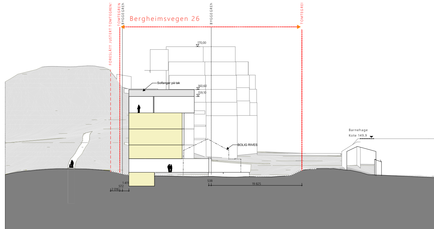
Snitt A-A
