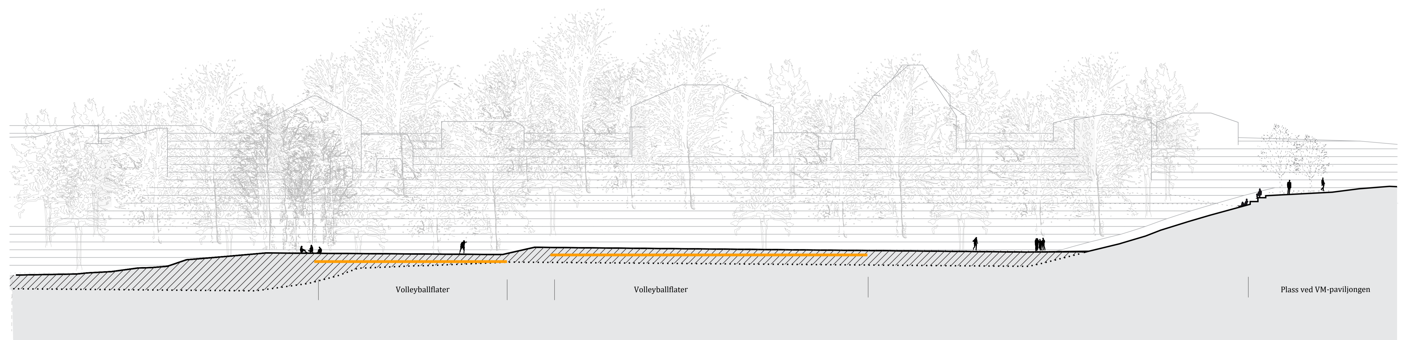
PRINSIPPSNITT KK Høgskoledalen II Fase 2
