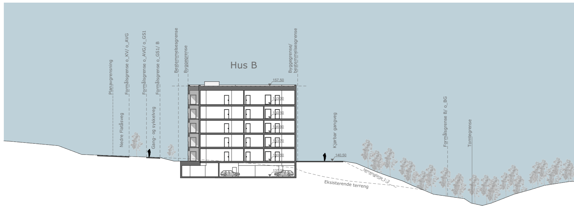
Snitt B-B
