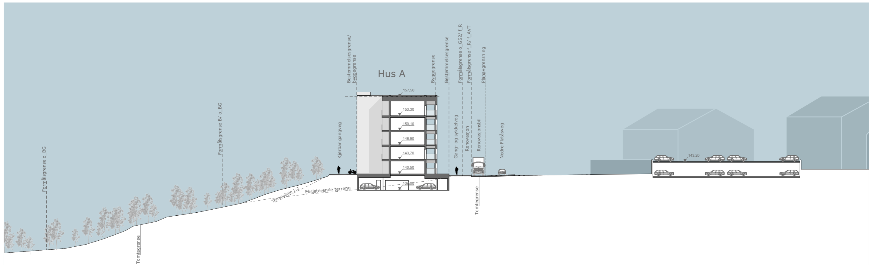
Snitt A-A
