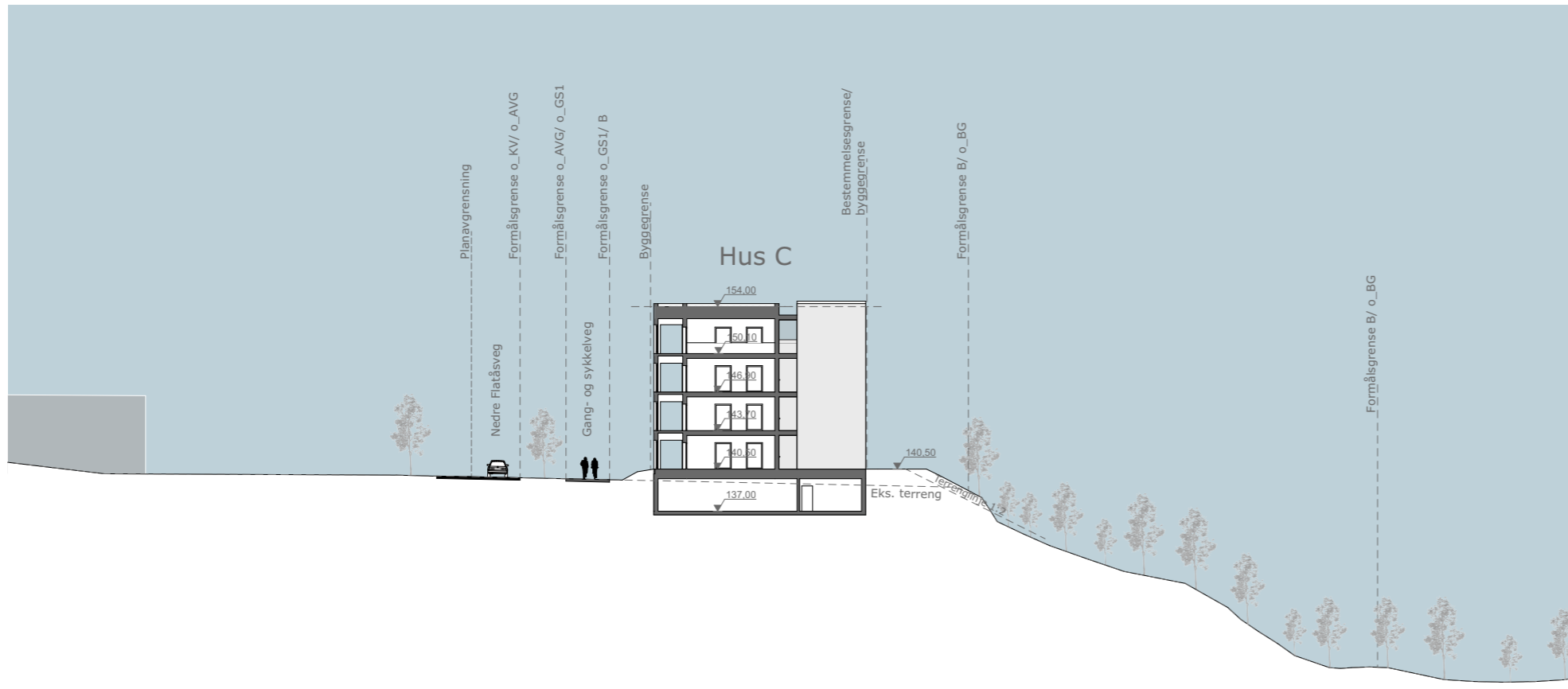
Snitt C-C
