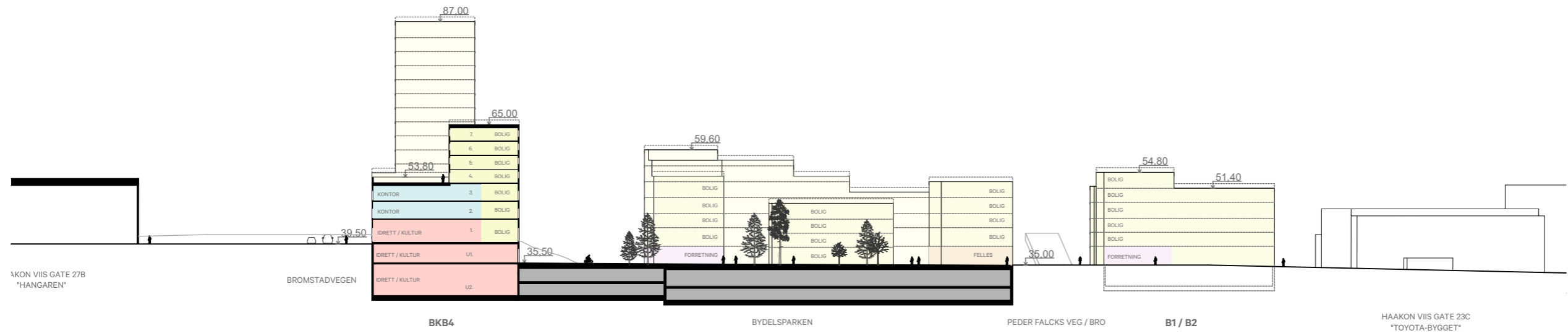
SNITT A-A: BKB4 & Bydelsparken (mot sør)
