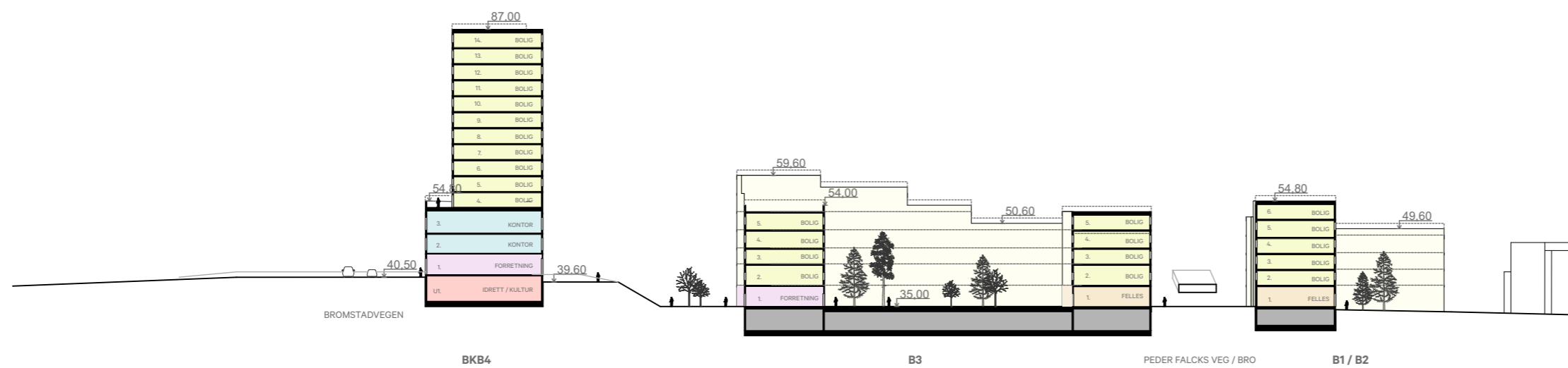
SNITT B-B: BKB4, B3 & B1/B2 (mot sør)
