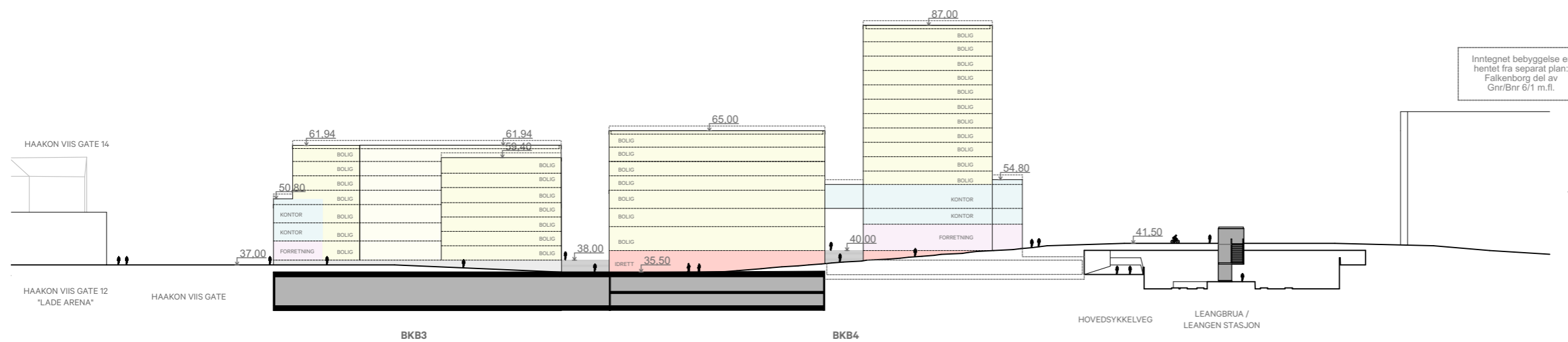
SNITT F-F: Gågate, bydelspark og utvidelse av Leangbrua (mot øst)
