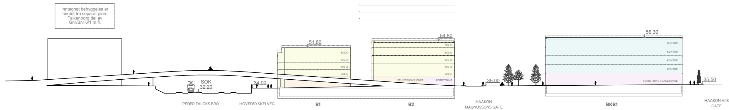
OPPRISS C: Peder Falcks veg (mot vest)
