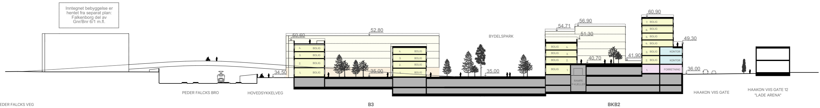
SNITT C-C: B3, bydelspark & BKB2 (mot vest)
