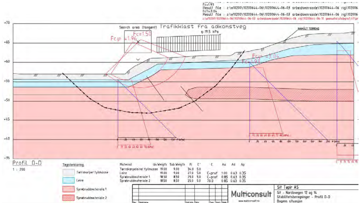
Figur 6: Utsnitt fra stabilitetsberegning for profil D, utført av Multiconsult [7]
