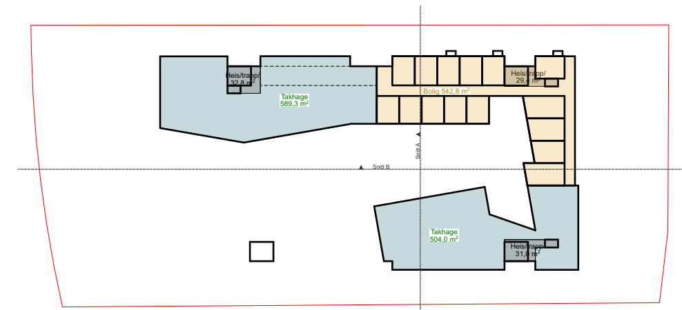
1:1000 7. Etasje
