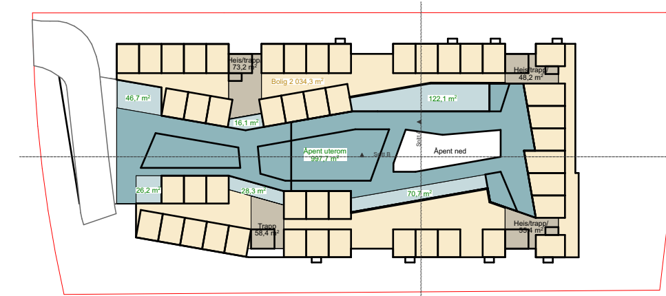
1:1000 3. Etasje
