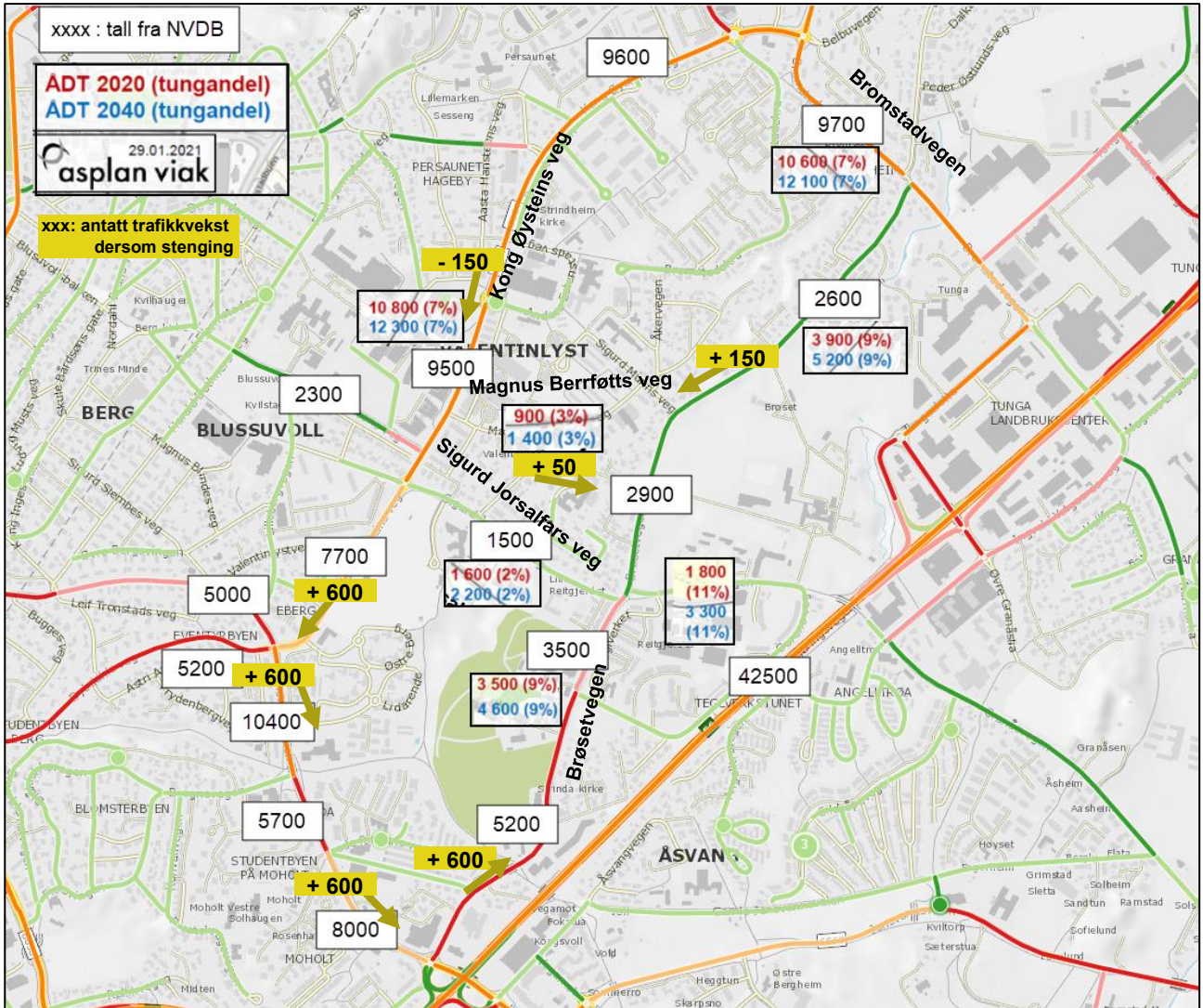
Figur 87: Anslag på dagens og fremtidige trafikkmengder på vegnettet omkring planområdet, ved envegsregulert Sigurd Jorsalfars veg.
