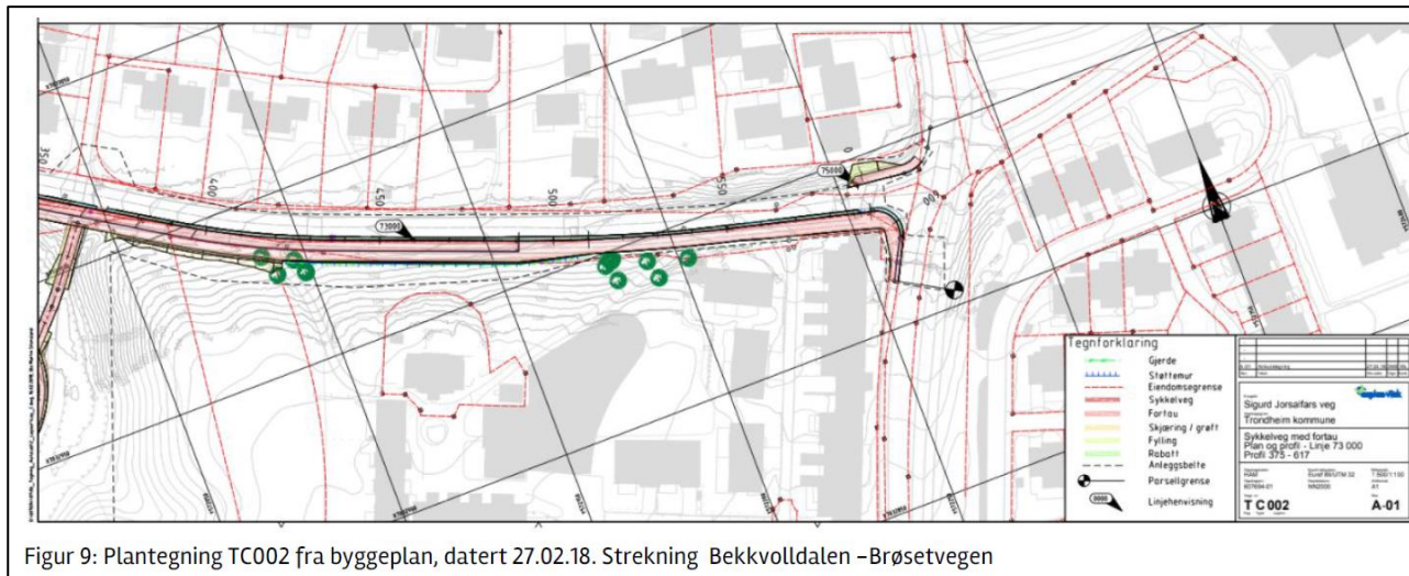
Figur 9: Plantegning fra byggeplan, Bekkvoll dalen - Brøsetvegen.
