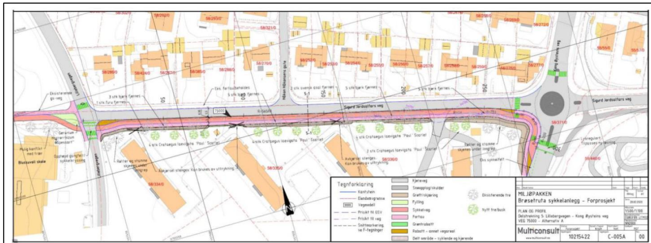
Figur 7: Lillebergvegen – Kong Øysteins veg, Plantegning C-005A fra forprosjekt for Brøsetruta, datert 28.02.2020
