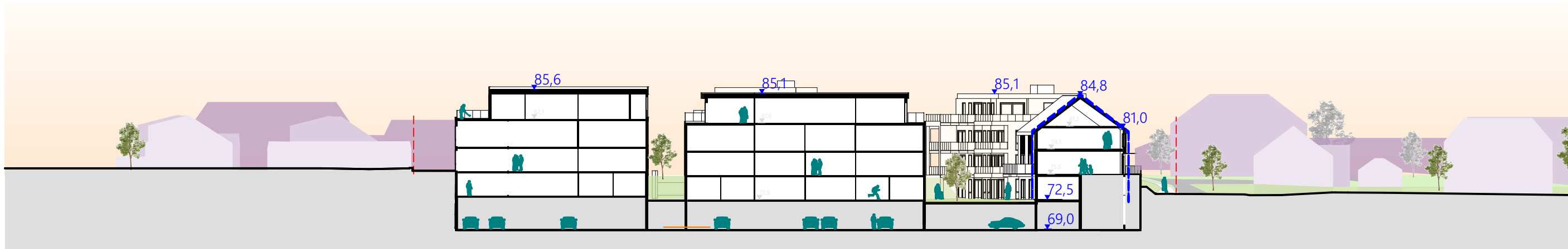
Snitt AA
