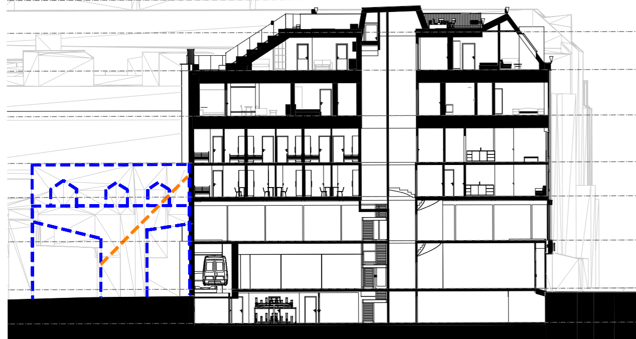
Snitt gjennom Jomfrugata 14 - planlagt status
