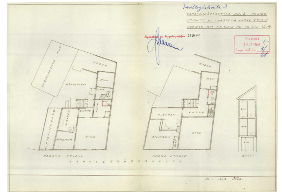
Plan og snitt fra Byarkivet
