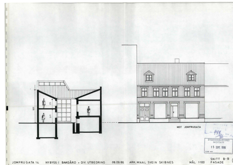
Snitt og fasade fra Byarkivet
