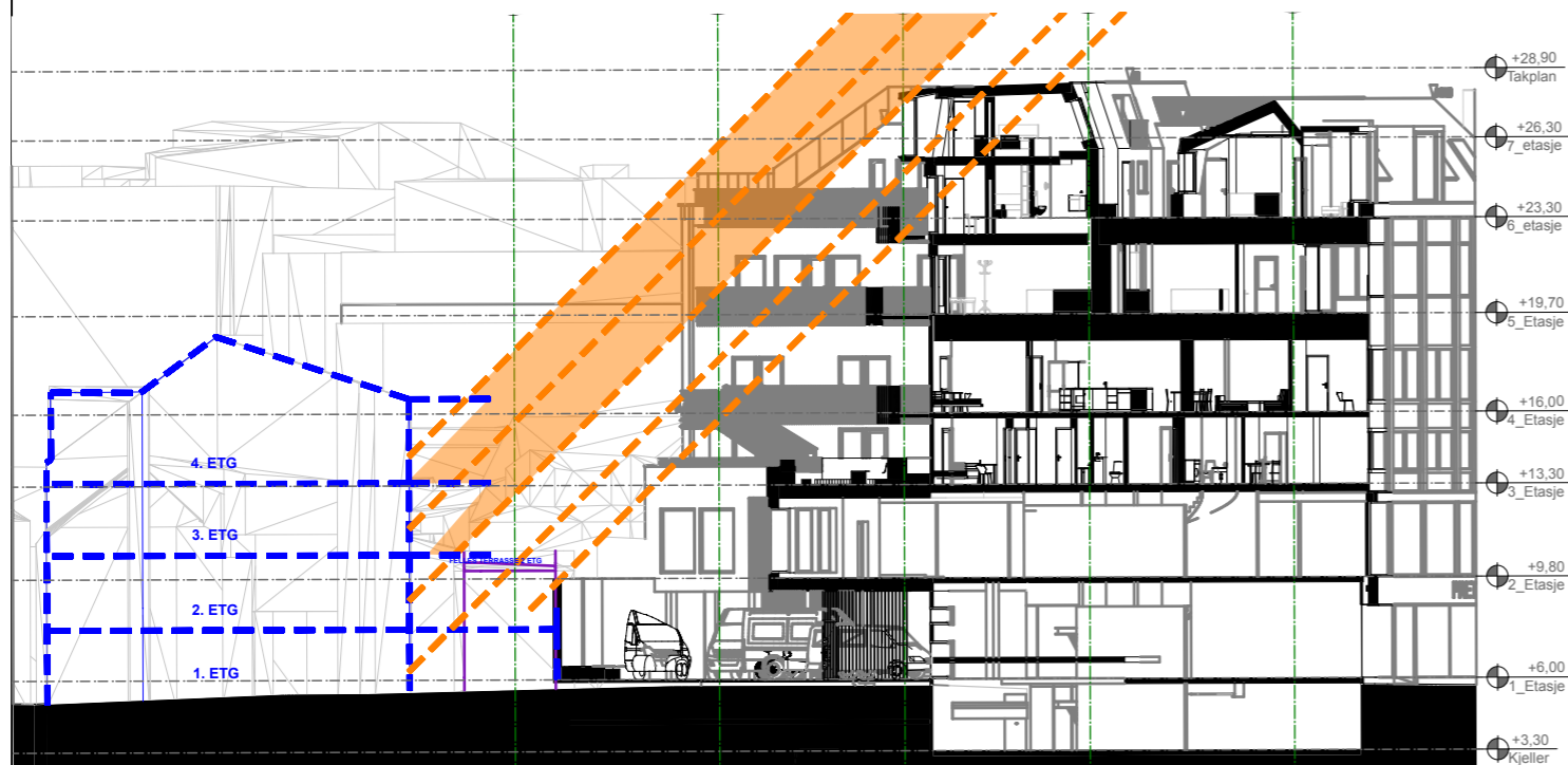
Snitt gjennom Taraldgårdsveita 7 - planlagt status
