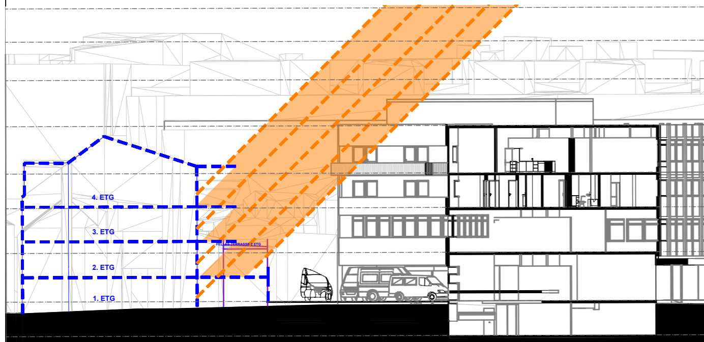
Snitt gjennom Taraldgårdsveita 7 - eksisterende status
