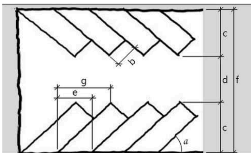
Figur 4.7.1.2–1 – Dimensjoner for tverrstilt parkering ved ulike vinkler.
