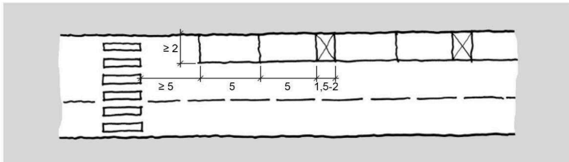
Figur 4.7.1.1—1 — Langsgående parkering (mål i m).
