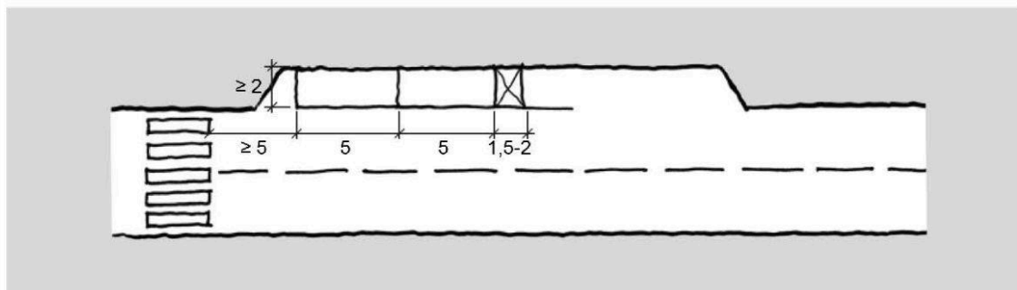
Figur 4.7.1.1—2 — Parkeringslomme (mål i m).
