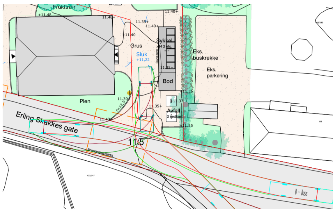
Utsnitt fra utomhusplanen viser to nedgravde containere og renovasjonsbilens ryggemanøver.
