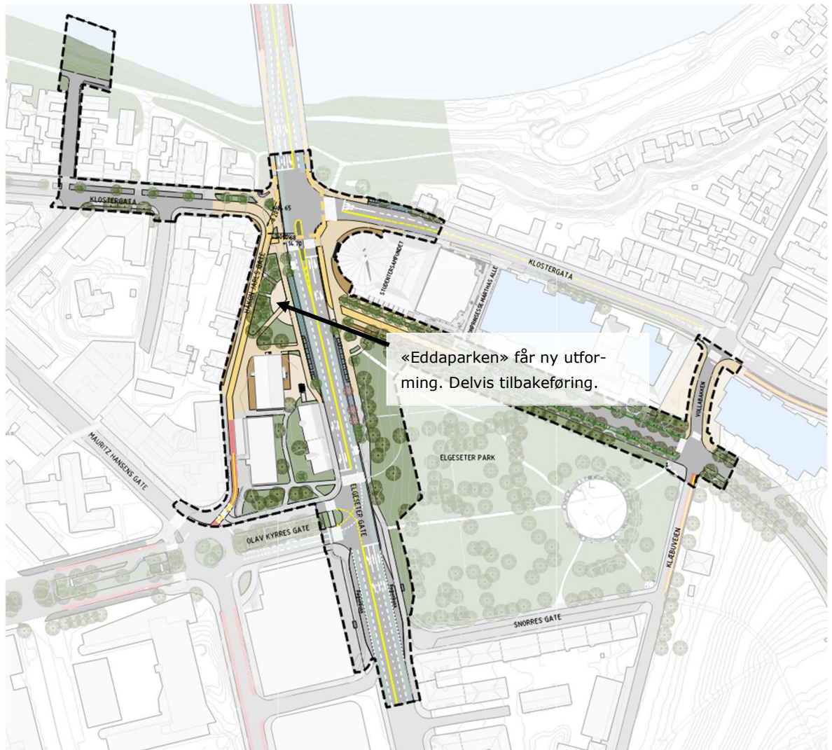
Figur 6-13: Utsnitt av illustrasjonsplan, datert 03.04.2025. Kilde: COWI AS.
