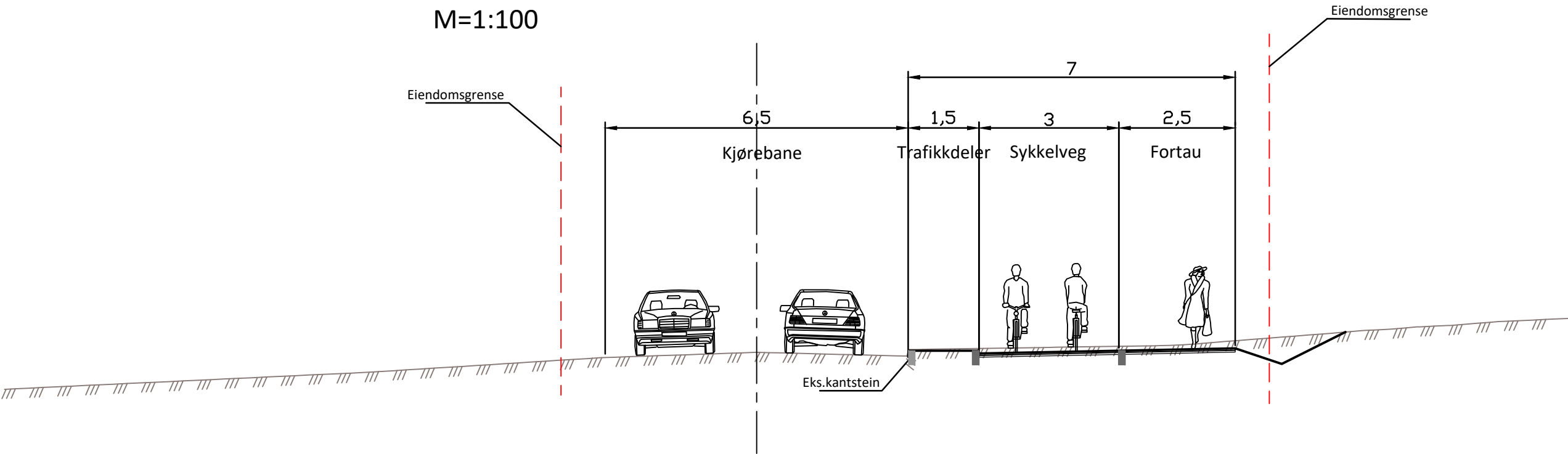
Granåsvegen, 2-feltsveg m/ 1,5 m trafikkdeler Profil 100-380 (snitt pr. 200) M=1:100
