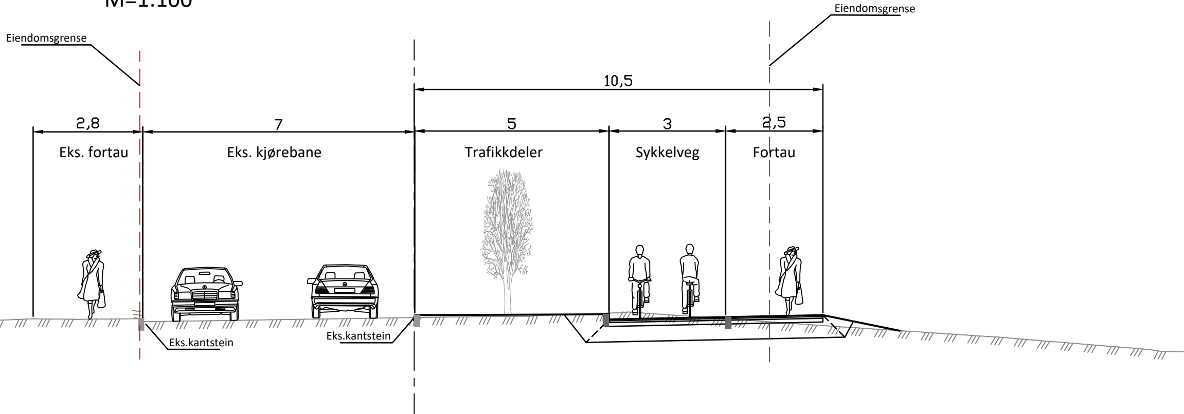
Tungasletta, sykkelveg med fortau langs eks. veg Profil 0-280 (snitt pr. 100) M=1:100
