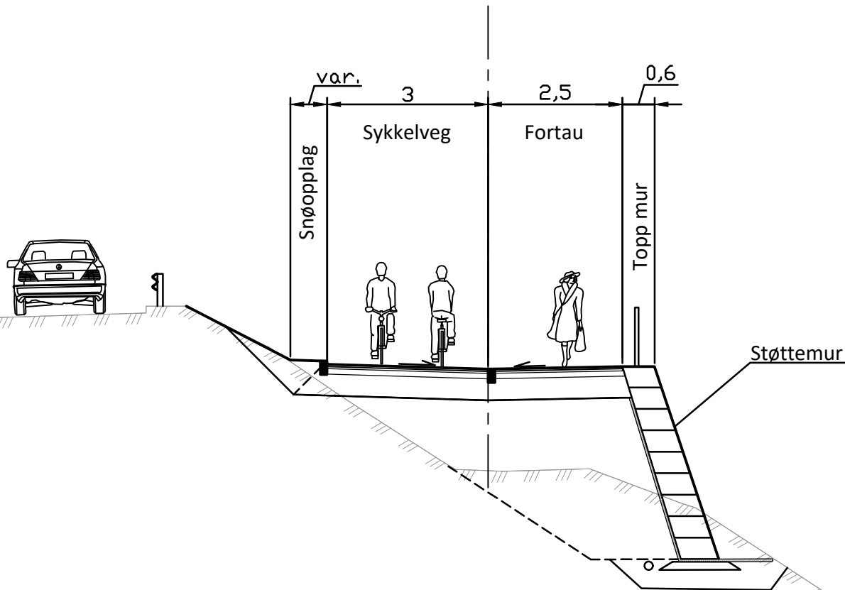
Sykkelveg med fortau, langs turdrag og gjennom Reitgjerdet kulvert Profil 0-450 (snitt pr. 77) M=1:100
