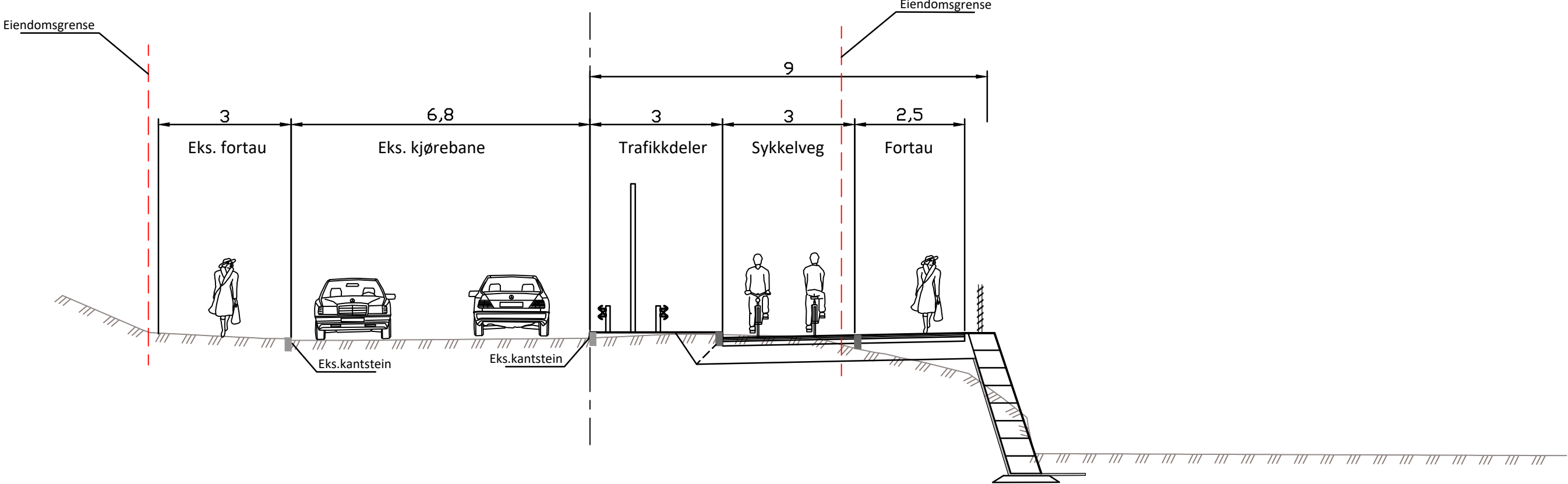
Tungasletta, sykkelveg med fortau langs eks. veg Profil 280-350 (snitt pr. 300) M=1:100
