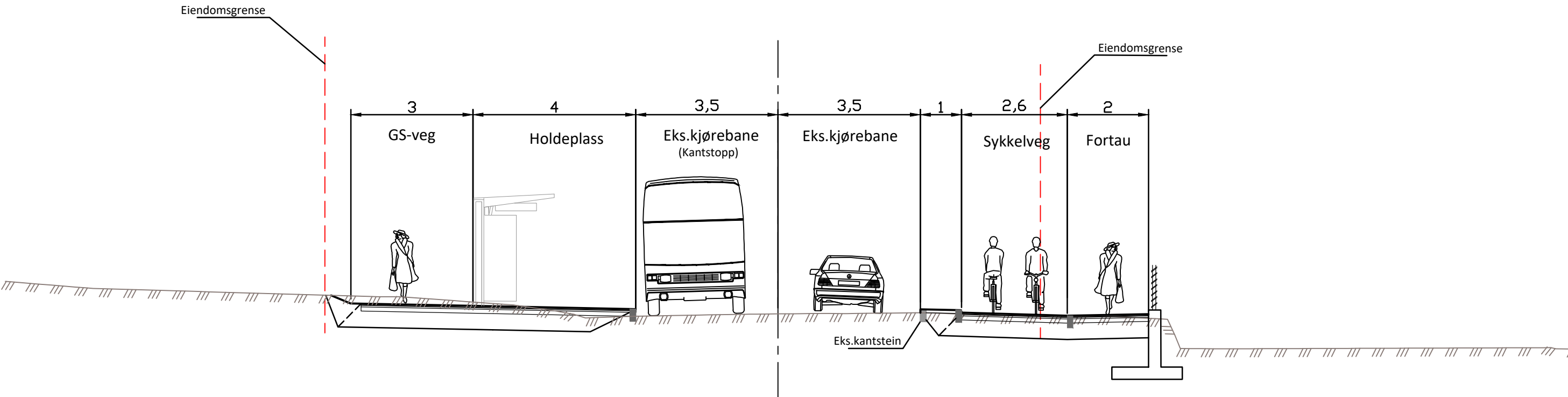
Ingvald Ystgaards veg, 2-feltsveg m/ 1 m trafikkdeler Profil 40 v/ holdeplass M=1:100
