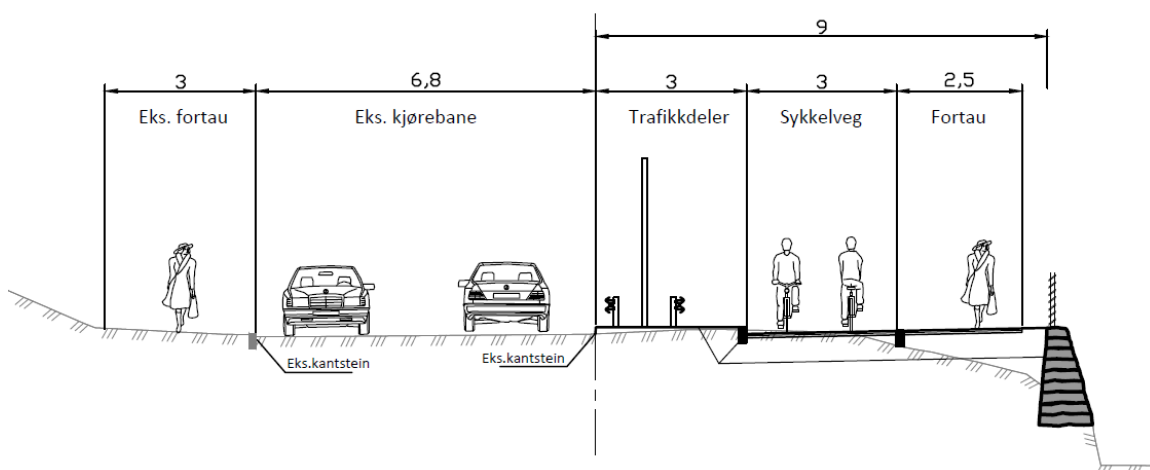
Figur 41: Tungasletta tverrsnitt ved dagens bomstasjon i trafikkdeleren og mur på yttersiden, profil 280-350
