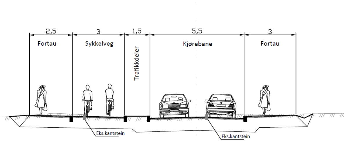
Figur 25: Normalprofil Bromstadekra, profil 0-140
