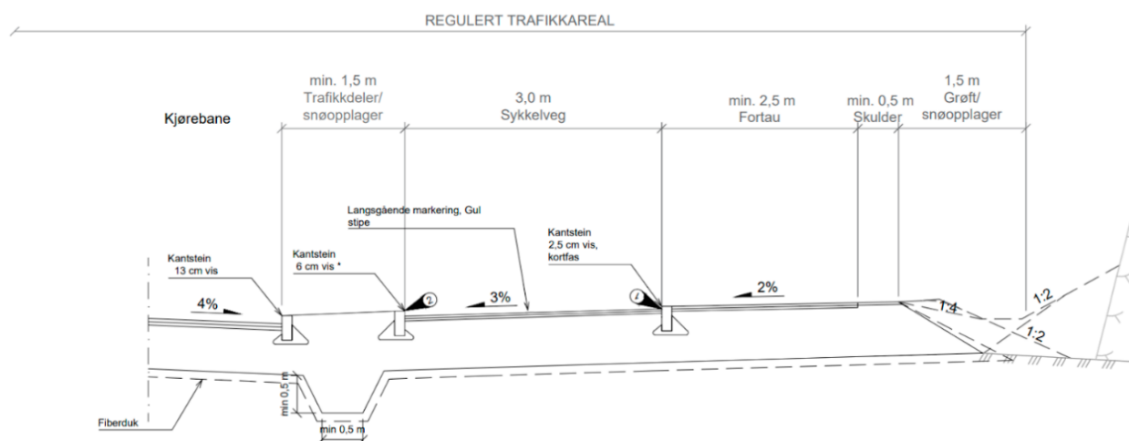
Dimensjonerende grunnlag for planlegging av sykkelveg med fortau. 3,0 m sykkelveg og 2,5 m fortau
