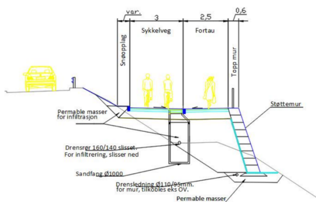
Forslag til tverrsnitt langs Brøsetdalen
