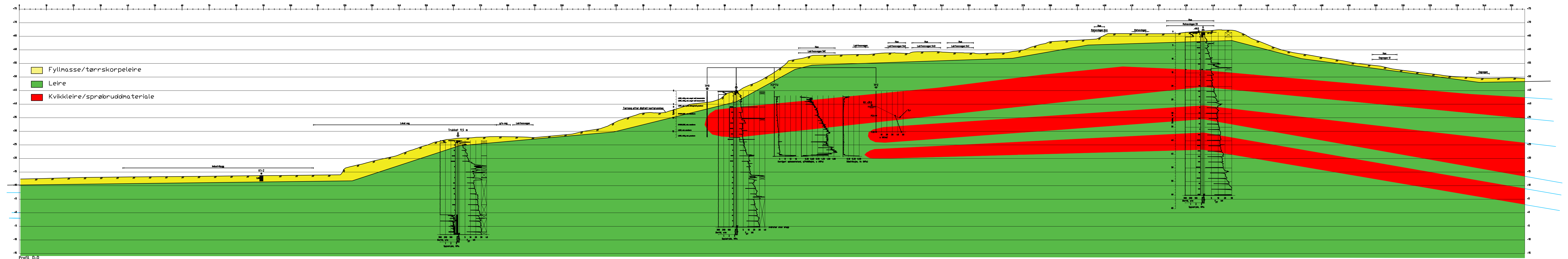
Profil D-D
