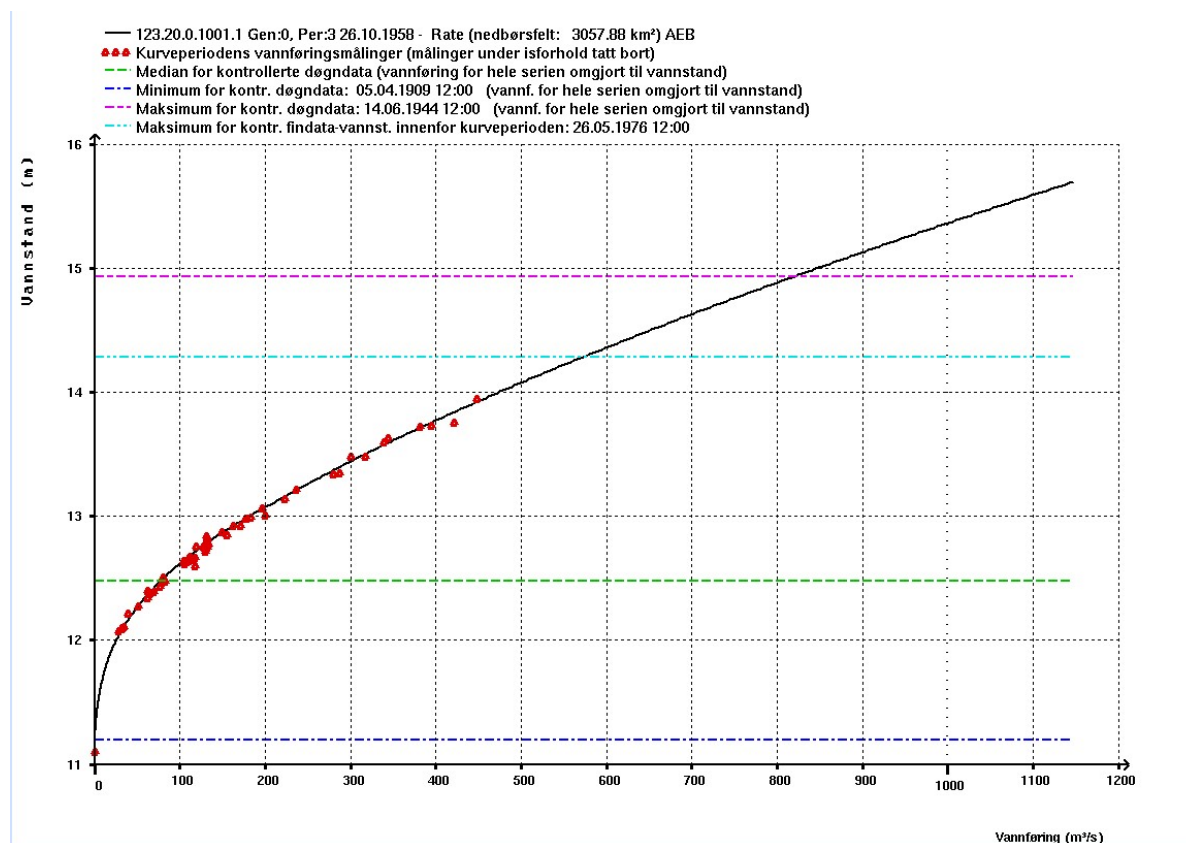
Figur 3-2: Vannføringskurve for 123.20 Rate, hentet fra HYDRA II
