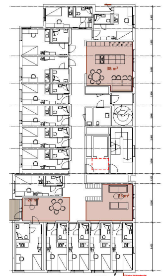
2. etasje
