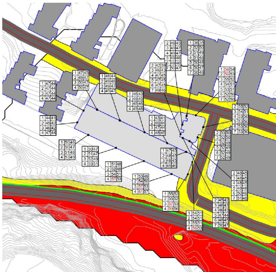
Figur 16 Støysonekart for vegtrafikk, modellert 1,5 meter over terreng, med forlengelse av skjerm langs Bynesvegen.
