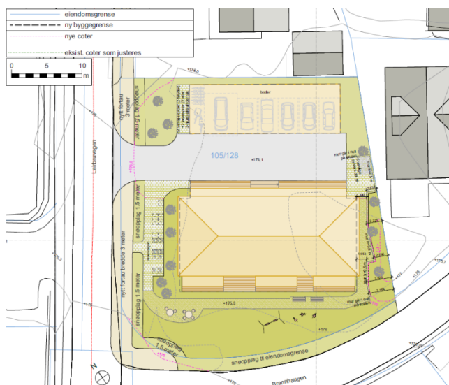
Terrengsnitt/oppriss sett fra sør og utomhusplan
