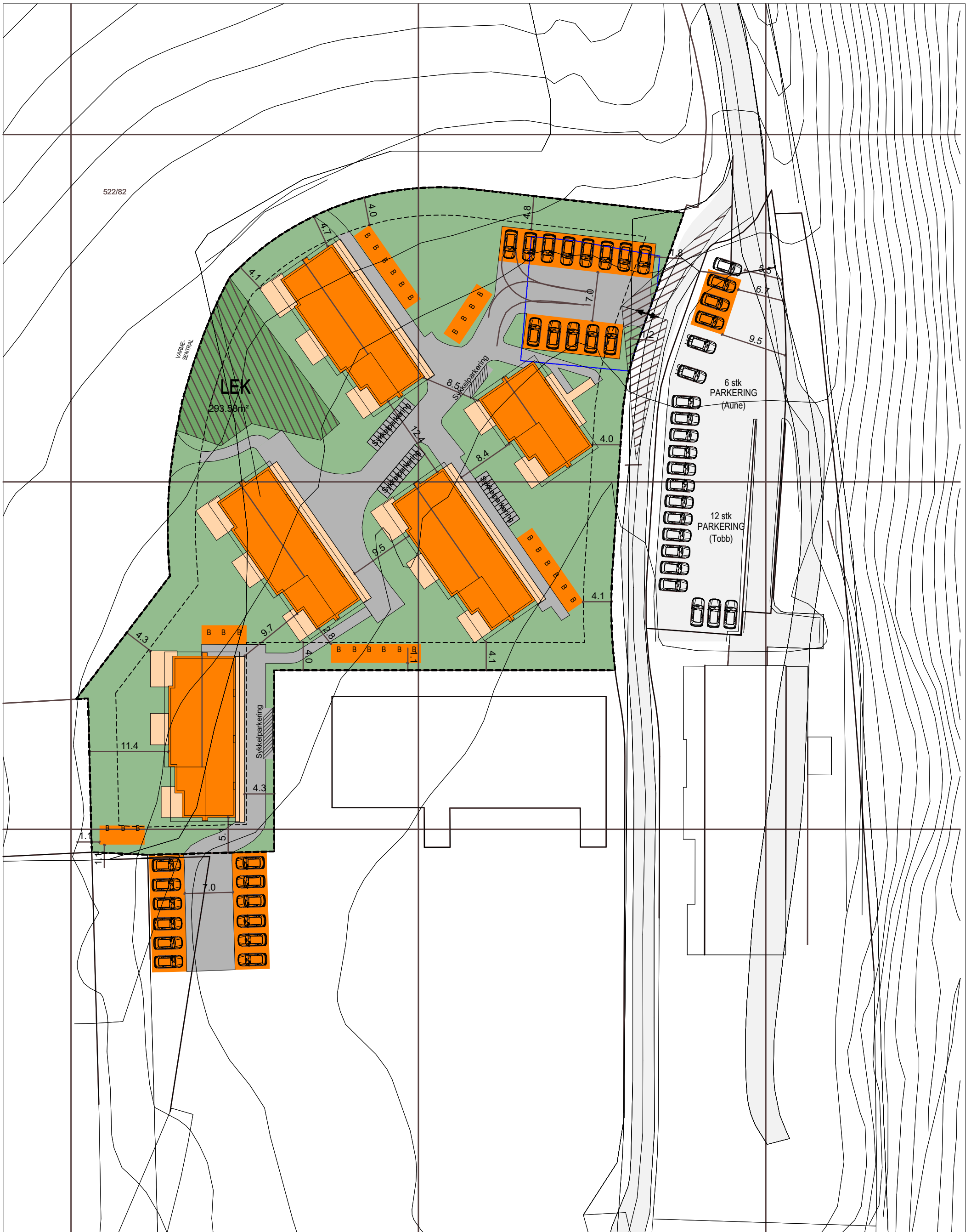
Situasjonsplan
